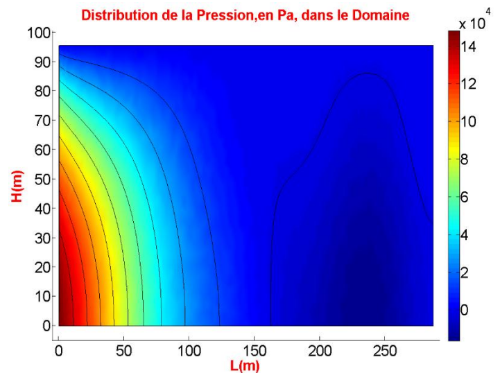
Fig. VIII.9 : La distribution de la pression, en Pa, dans le réservoir (MATLAB)
