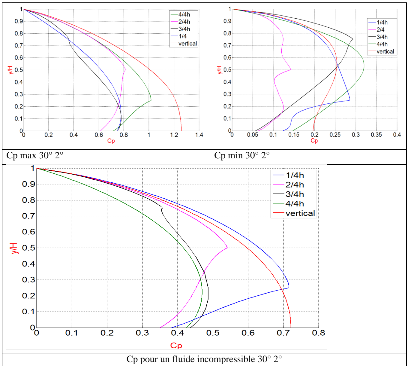
Fig.VI.28 : comparaison de la variation du coefficient de pression en fonction du rapport y/H pour différentes fractions de la hauteur incliné h pour une \beta=30^\circ et Gama=2^\circ .
