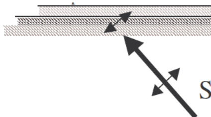
Fig.II.9 : l'onde S. [RIS]
