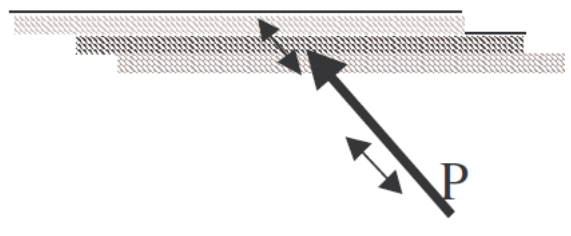
Fig.II.10 l'onde P. [RIS]
