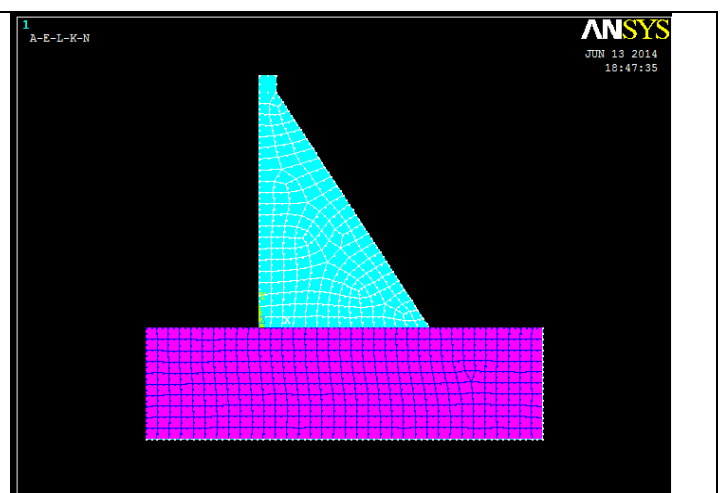
Fig. VIII.12 : Maillage du domaine sol-structure.
