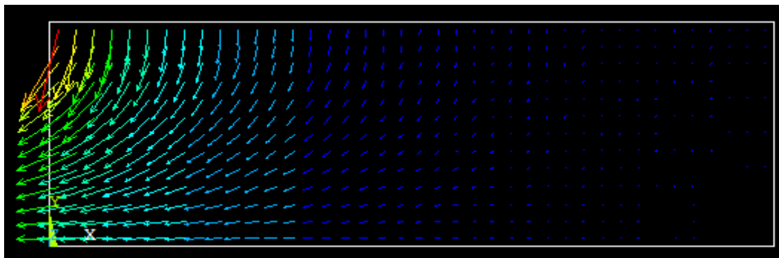
Fig. VIII.10 : La distribution de vecteur du gradient de la pression dans le Domaine
