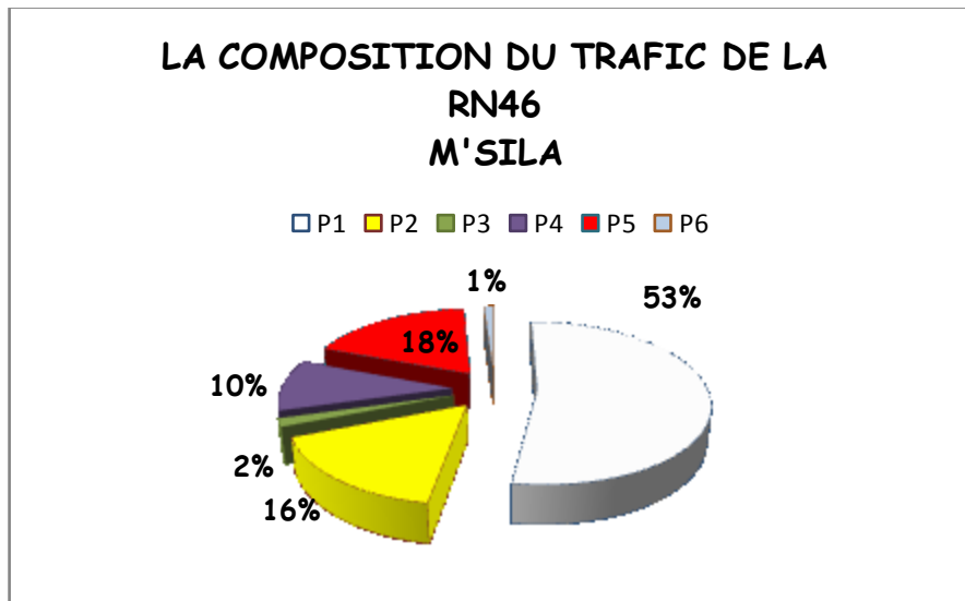
Figure III. 1 : La composition du trafic du la RN46 M'sila [3]
