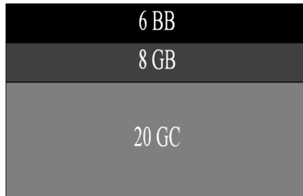
Figure IV. 6 : Structure de dimensionnement par la méthode CBR
