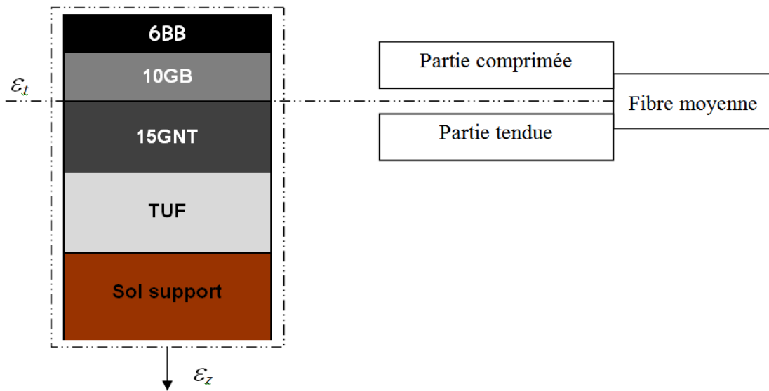
Figure IV. 10 : Modernisation de la 2 ème section
