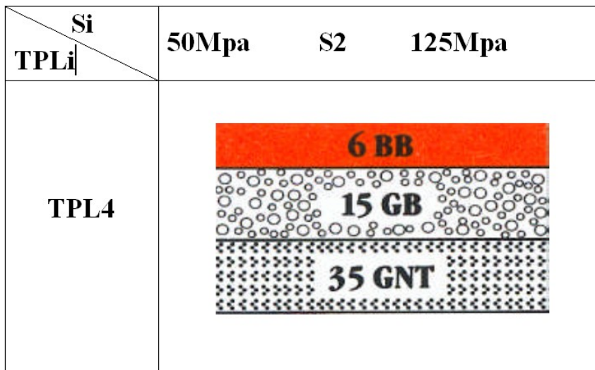
Figure IV. 7 : Structure de dimensionnement par la méthode du catalogue [5]
