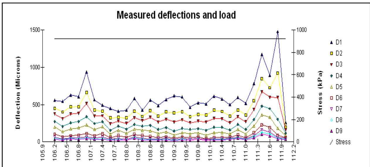
Figure III. 3 : Déflexions mesurées le long de la deuxième section homogène « SH2 » [9]
