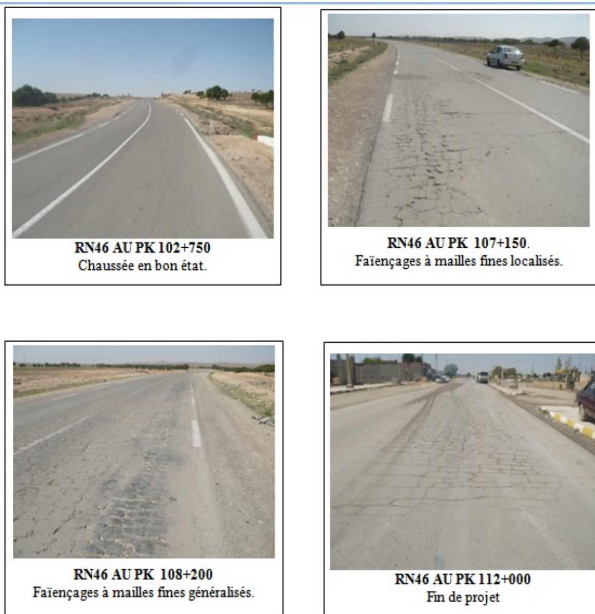
Figure III. 4 : photo des différentes dégradations [3]
