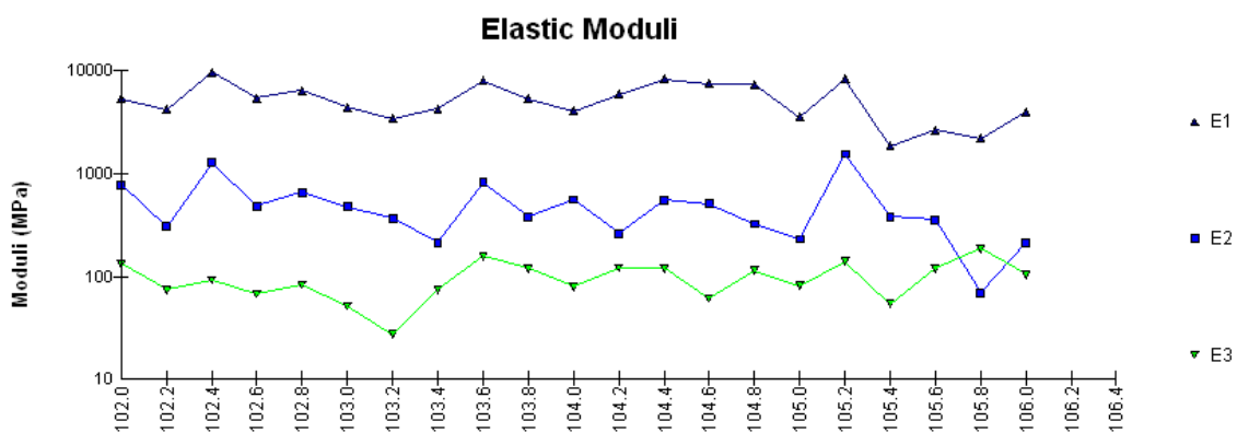
Figure IV. 2 : Les modules d'élasticités résiduels des différentes couches de la chaussées de la section « SH1 » [9]
