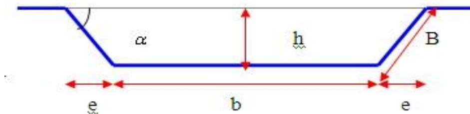
Figure v. 1 : profil en travers hypothétique de fossé [2]
