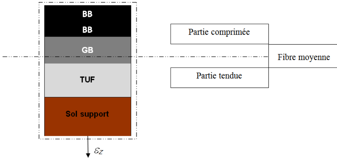
Figure IV. 9 : Modernisation de la 1 ère section
