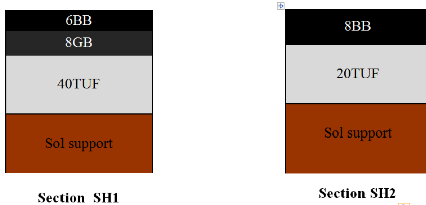
Figure IV. 1 : Structures des chaussées existantes [3]
