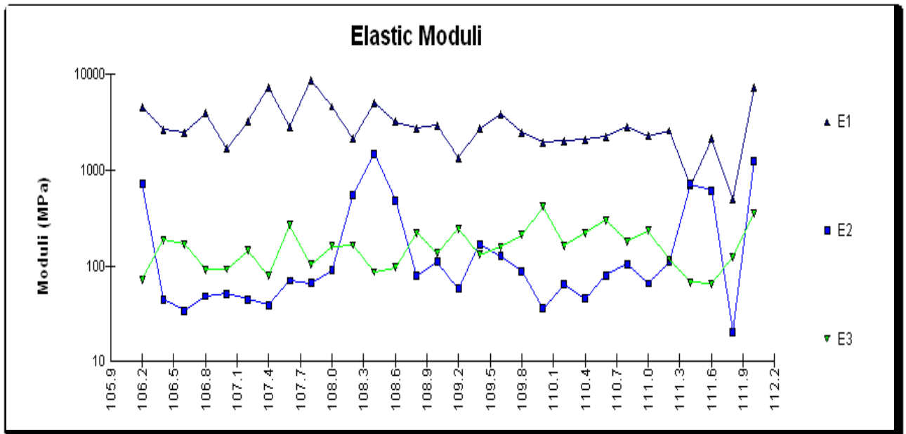
Figure IV. 3 : Modules d'élasticités des différentes couches de la chaussée de la section « SH2 » [9]
