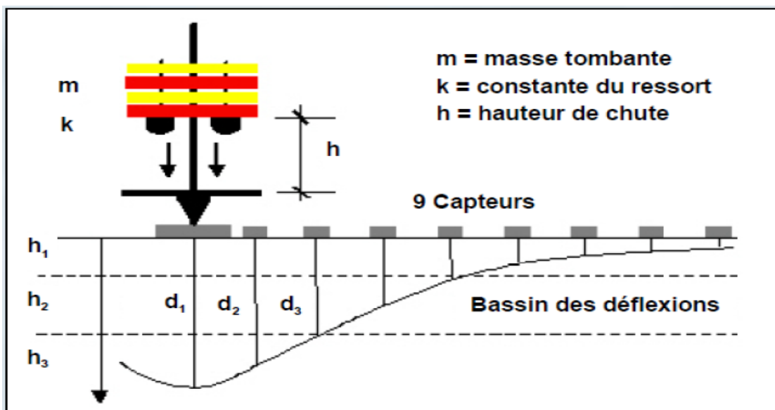
Figure II. 4 : Le bassin de déflexion [3]
