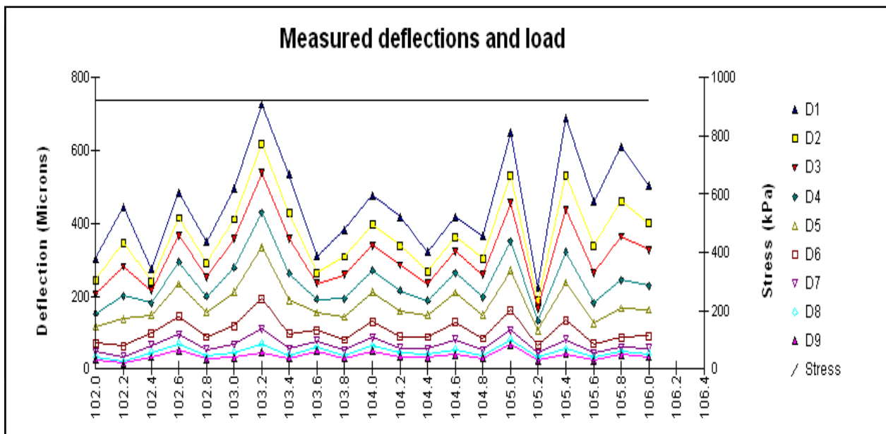
Figure III. 2 : Déflexions mesurées le long de la première section homogène « SH1 » [9]
