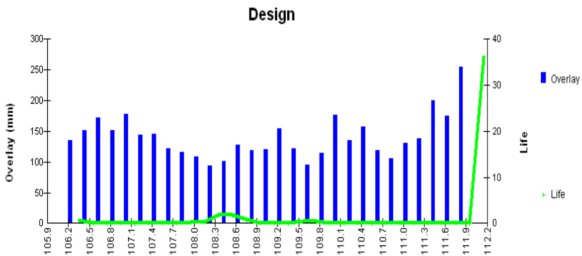
Figure IV. 5 : Durée de vie et épaisseur de renforcement de la « SH2 » [9]
