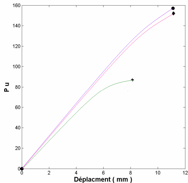
Figure 3.12 : Courbe charge – flèche pour les poutres rompues par traction diagonale
