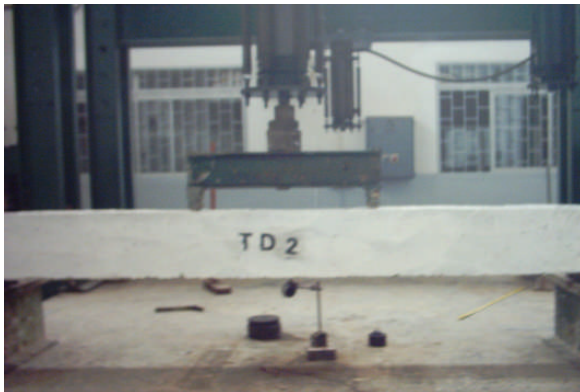
Figure 8 : Poutres témoins en cour du chargement
